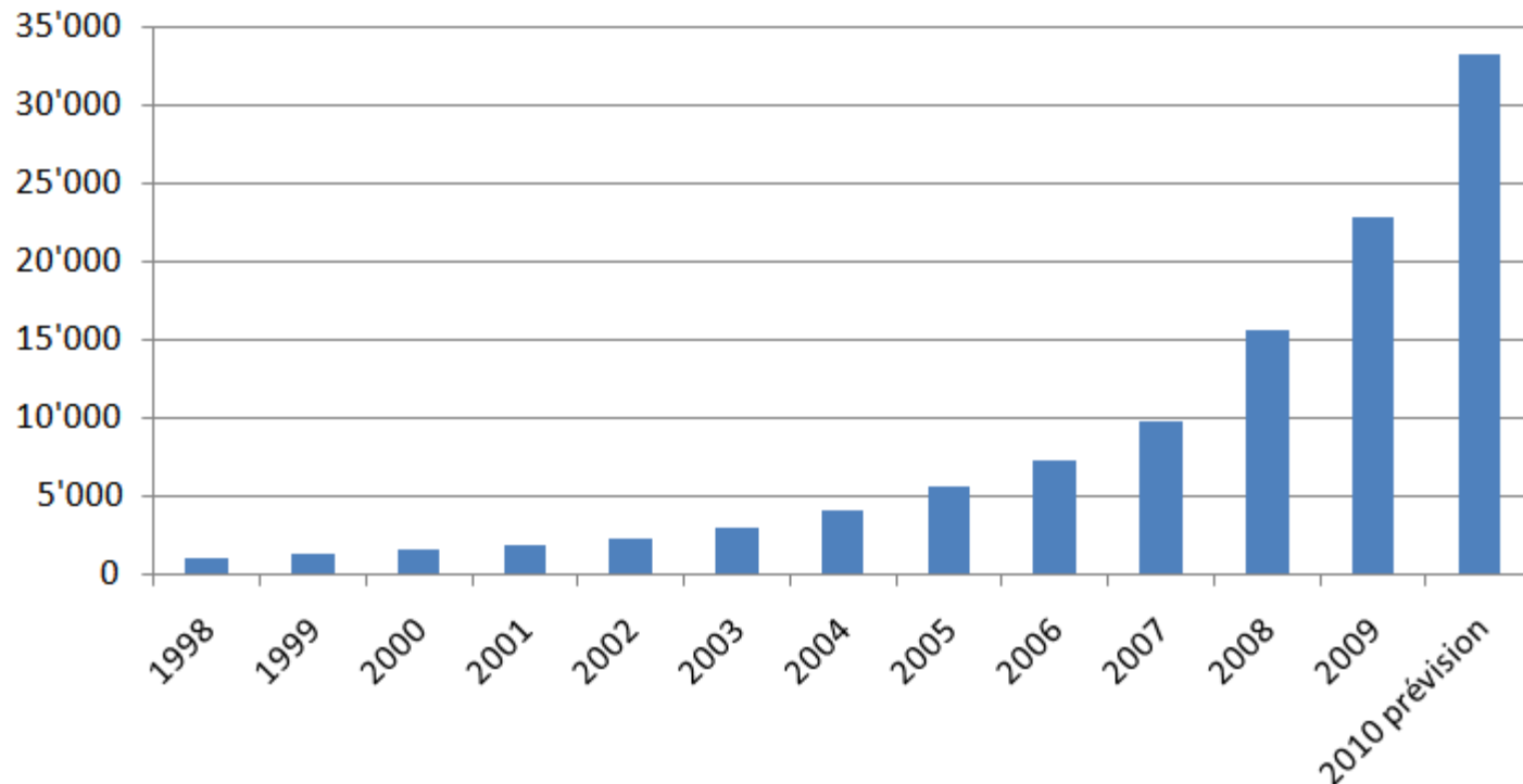
MW Photovoltaïque (puissance de crête)
